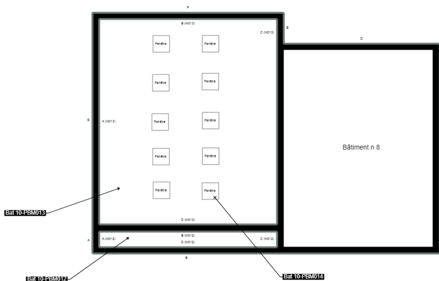
Pignon droit du bâtiment n 10
